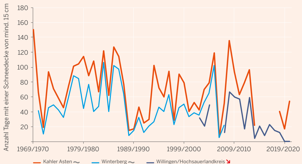
Abb. 124: Anzahl von Tagen mit einer Schneedecke von mindestens 15 cm während des Winters (November - April) an insgesamt drei Beobachtungsstationen im Sauerland um Winterberg und Schmallebenberg herum von 580 m bis 838 m ü. NN im Zeitraum 1969/1970 - 2020/2021 (Datengrundlage: DWD)
