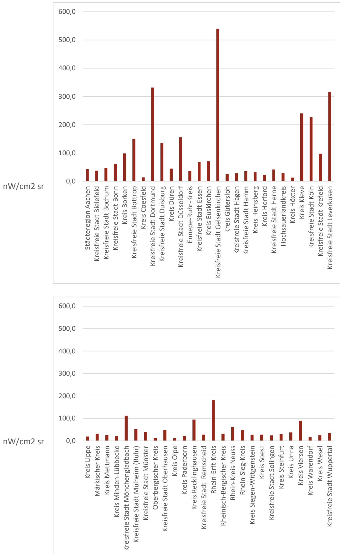
Abbildung 13: Diagrammdarstellung der Maximalwerte der Strahlungsintensität („größte Helligkeit“) aus Tabelle 1
