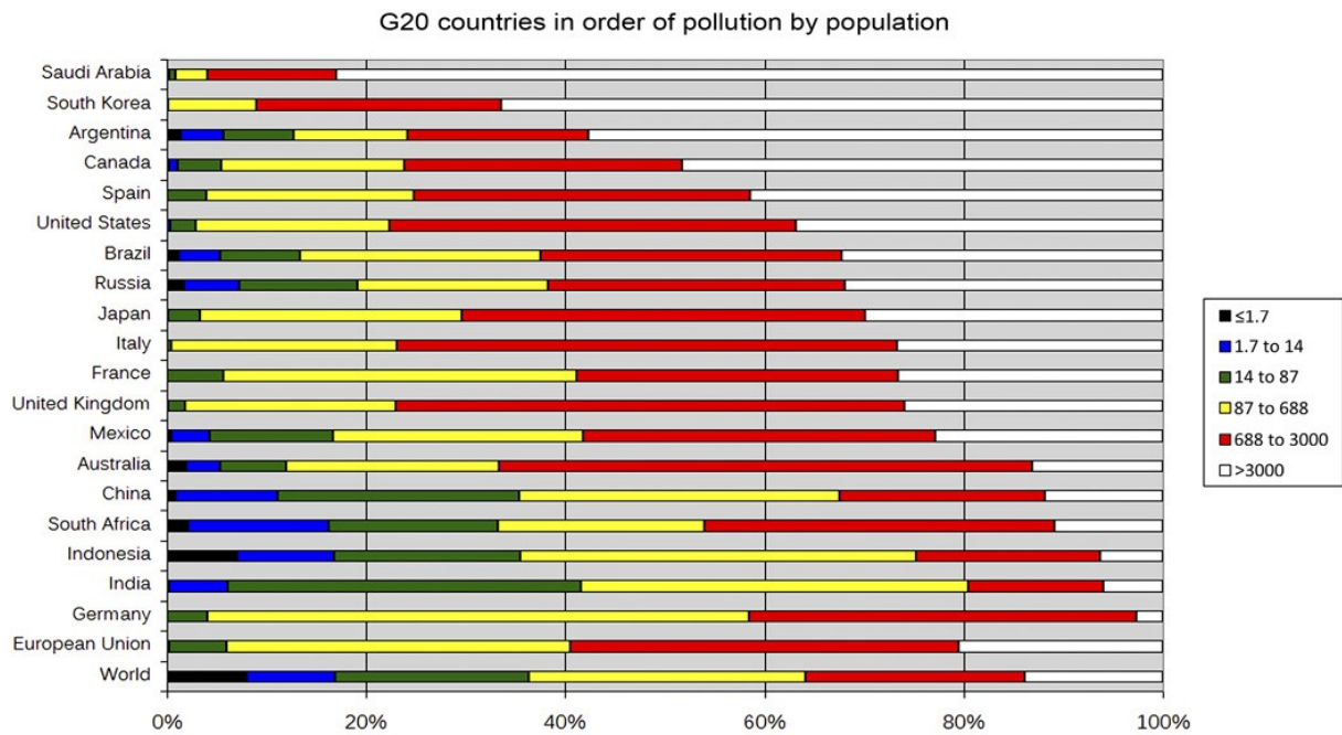
Abbildung 5: G20-Länder. Prozentuale Anteile der Bevölkerung nach dem Niveau der Lichtverschmutzung; Auflistung nach dem Bevölkerungsanteil mit dem am höchsten durch Lichtverschmutzung exponierten Niveau (Angaben in \mu\text{cd}/\text{qm} ) © F. Falchi et al [65]
