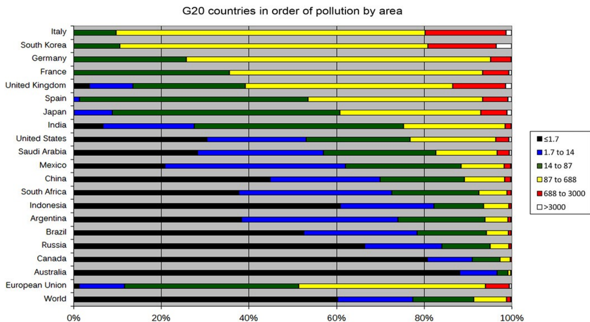
Abbildung 6: G20-Länder. Prozentuale Anteile der Landesfläche nach dem Niveau der Lichtverschmutzung; Auflistung nach den flächenmäßig am meisten lichtverschmutzten Ländern (Summe weiß, rot, gelb; Angaben in \mu\text{cd}/\text{qm} ) © F. Falchi et al [65]
