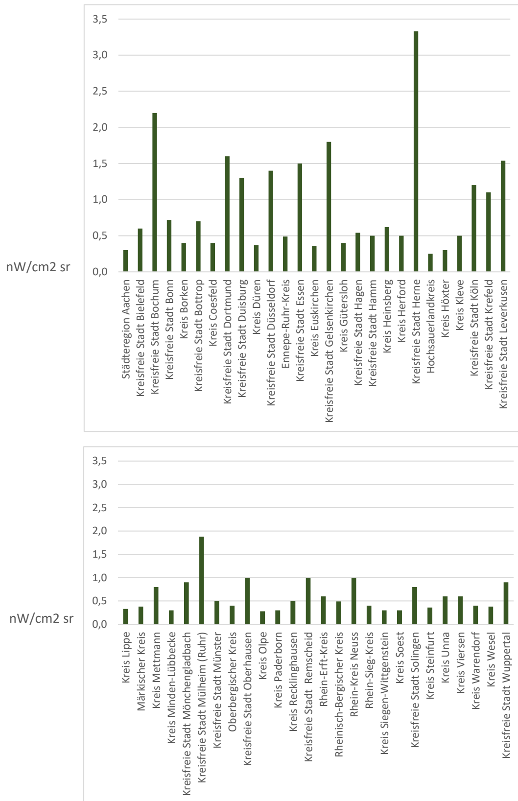
Abbildung 11: Diagrammdarstellung der Minimalwerte der Strahlungsintensität im Kreisgebiet („geringste Helligkeit“) aus Tabelle 1
